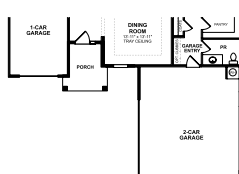
OPTIONAL ELEVATION F
