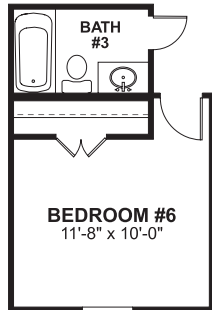
OPTIONAL BEDROOM #6/ BATH #3
