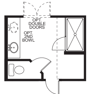
OPTIONAL ENCLOSED TOILET
