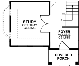
OPTIONAL STUDY
