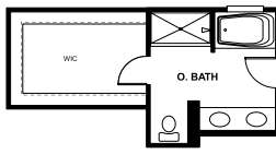
OPTIONAL DELUXE BATH
