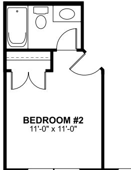
OPTIONAL BATH 3
