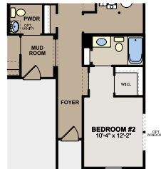
OPTIONAL BEDROOM #2 BATH
